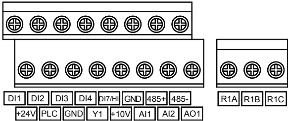
Рис. 3-9 Клеммы цепи управления Таблица 3-4 Описание клемм цепи управления FR150
