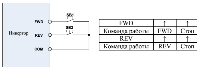
Рисунок 6-12 Схема управления импульсной операцией останова
