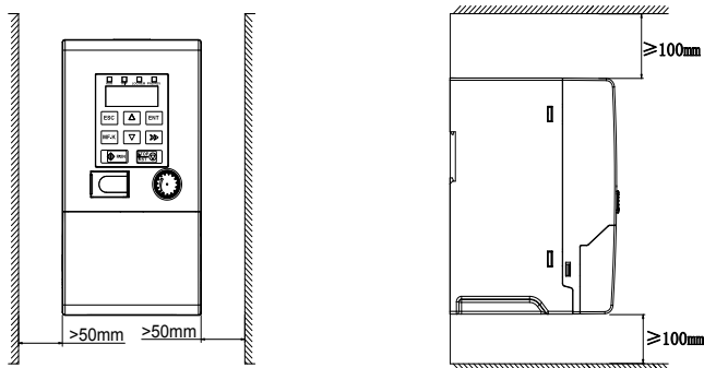
Рис. 3-1 Методы установки
