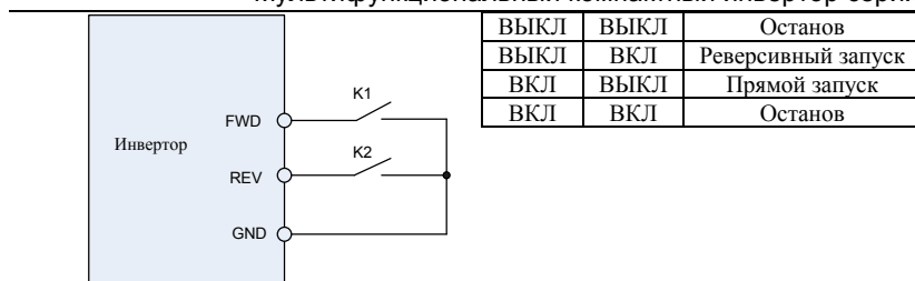
Рисунок 6-8 Установка двухпроводного режима 1
