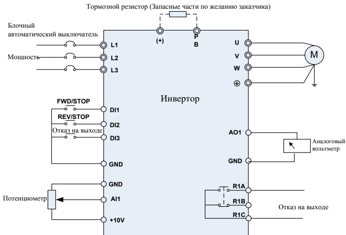
Рисунок 6 Объединенная схема
