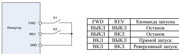
Рисунок 6-9 Установка двухпроводного режима 2
