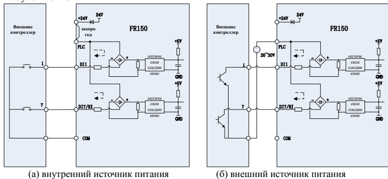
Рис. 3-11 Сухой контакт
