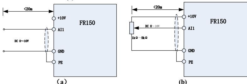
Рис. 3-10 Схема подключения вывода аналогового входа
