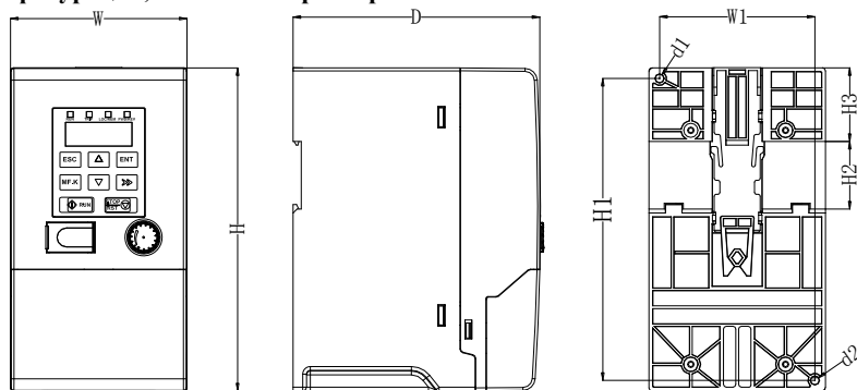
Fig 2-4 Габариты клавиатуры
