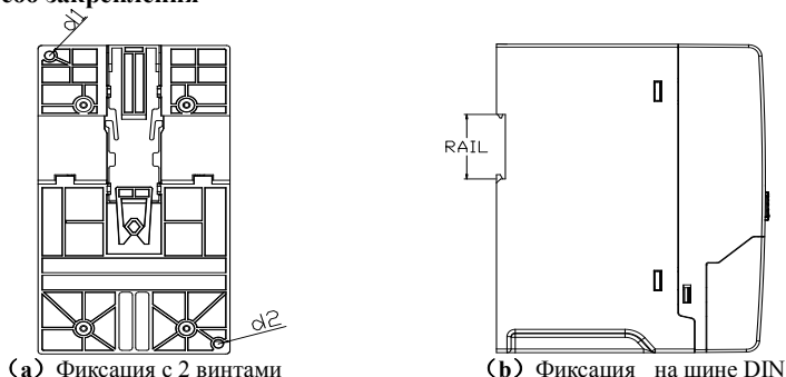
Рис. 3-2 Крепление
