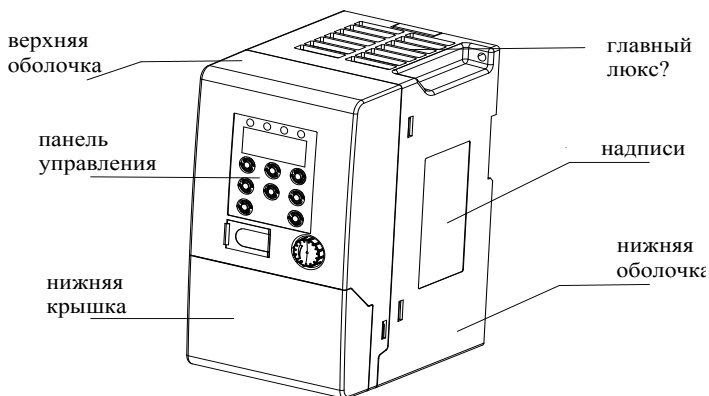
Рис. 2-3 Пример компоновки
