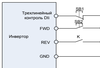
Рисунок 6-11 Настройка трехпроводного управления 2
