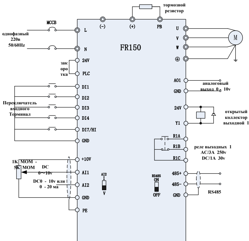
Рис. 3-5 Монтажная схема однофазного преобразователя 220 В
